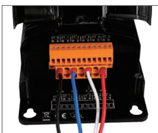
iWSN-9603 Wiring
