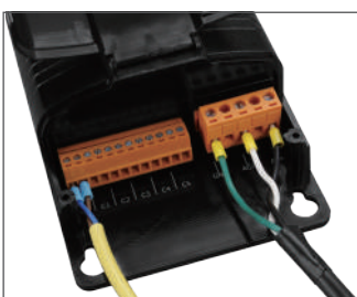
iWSN-9601 Wiring
